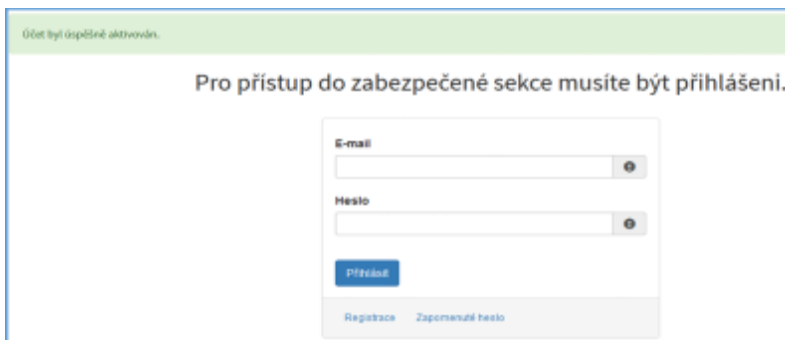
Obrázek 5 - Přihlášení
