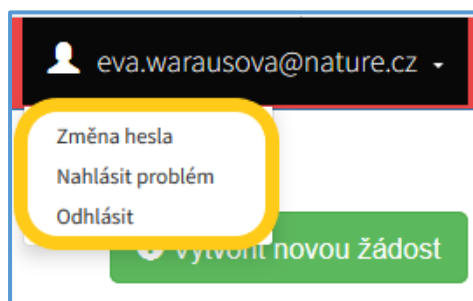
Obrázek 8 – nabídka funkcí
