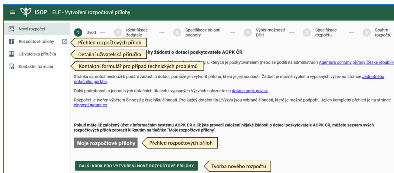
Obrázek 34 : Krok 1 - Úvod
